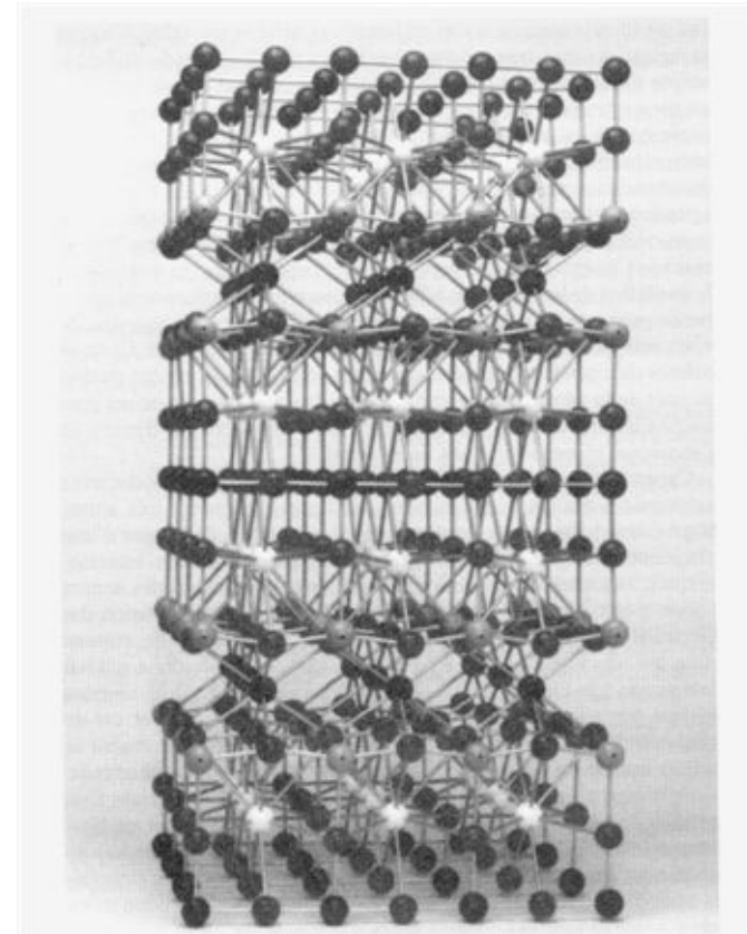
Structure pérovskite de \text{YBa}_2\text{Cu}_3\text{O}_7 (YBACUO) déficiente en oxygène. En gris clair : oxygène ; en gris foncé : cuivre ; en blanc : baryum ; en noir : yttrium (Laboratoire des solides irradiés, CEA / École polytechnique.)
